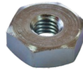
7587 PORCA DE APERTO DA BARRA EAN 5604547063877 M8 x 1,25 SEXTAVADO 19mm ADAPTÁVEL STIHL PACK 10
